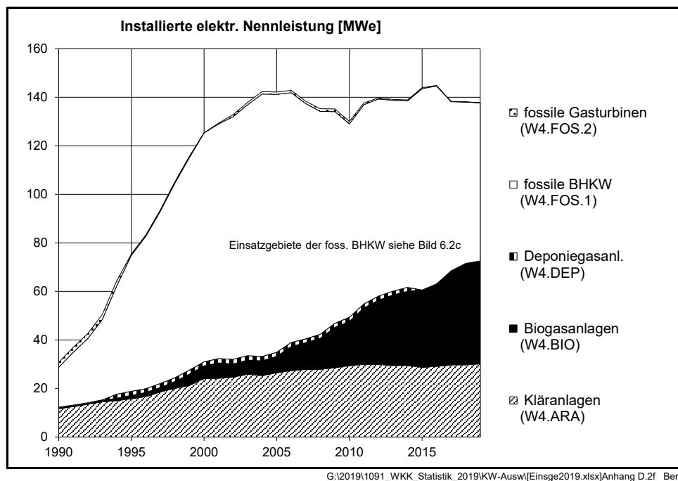
Bild 6.2b Entwicklung der elektrischen Nennleistungen der Klein-WKK-Anlagen nach Anlagekategorien
