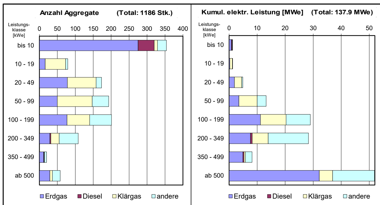
Bild 6.1f Ende 2019 in Betrieb stehende Klein-WKK-Aggregate, geordnet nach Leistungsklassen und nach Energieträgern
