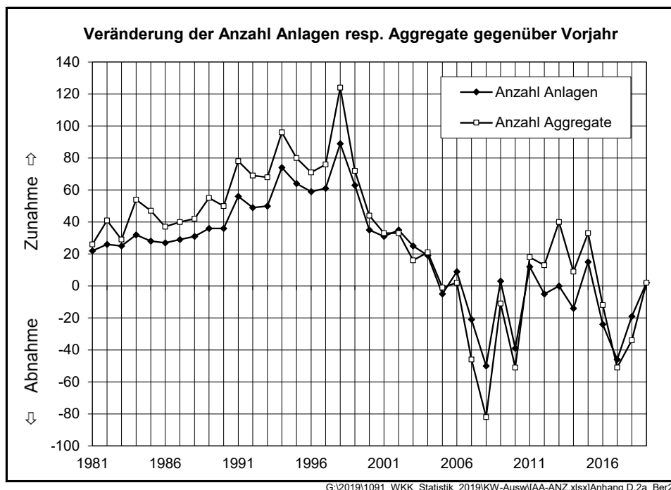
Bild 6.1a Jährliche Veränderung des Klein-WKK-Bestandes (siehe Anhang D.2a)
