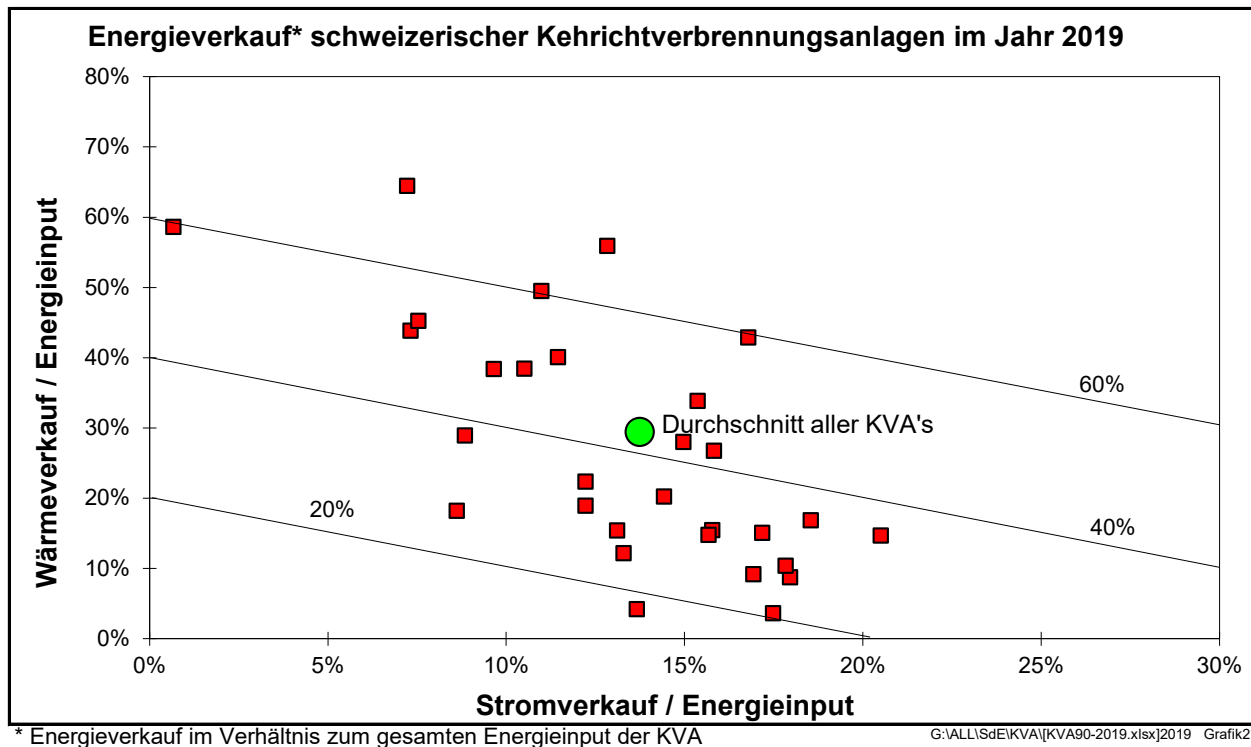
Bild 7.1d Energieverkaufs-Benchmark schweizerischer KVA (Jahr 2019)
