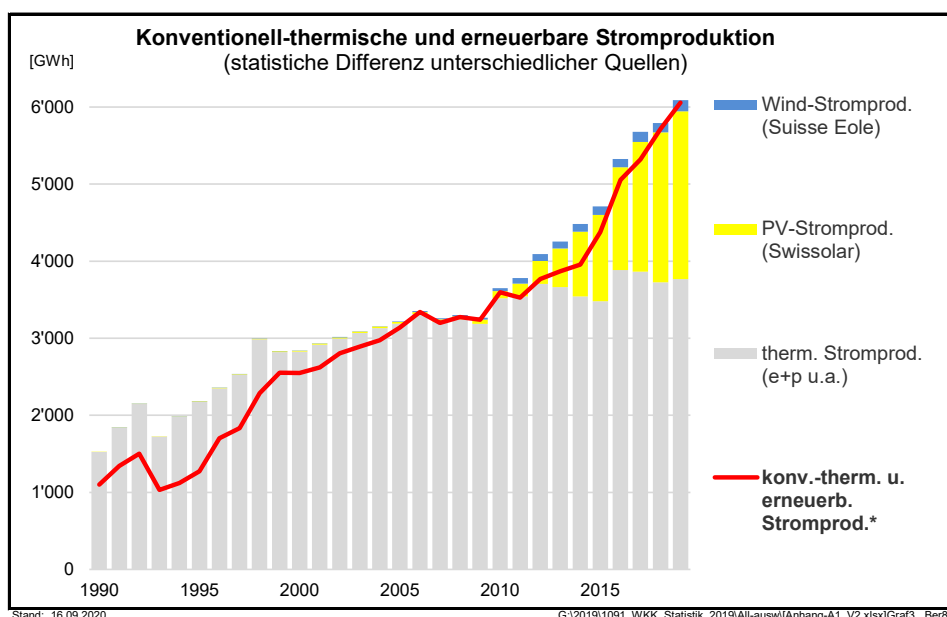
Bild 3.2b Stromproduktion „thermisch und andere“: Vergleich der schweizerischen Elektrizitätsstatistik (rot) mit den Erhebungen von e+p, Swissolar und Suisse Eole (Balken)
