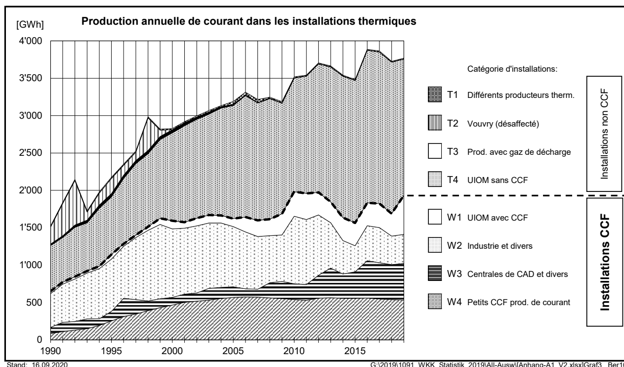
Figure 1.3 Evolution de la production thermique de courant
