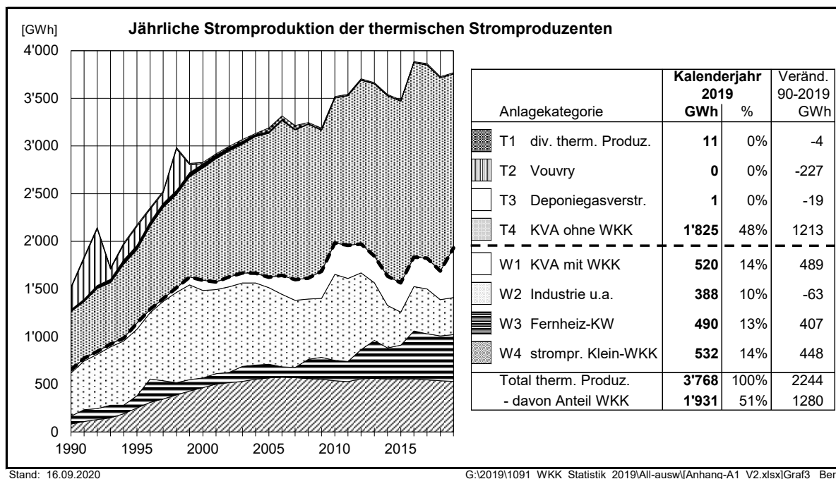
Bild 3.2a Thermische Stromproduktion der Jahre 1990 bis 2019
