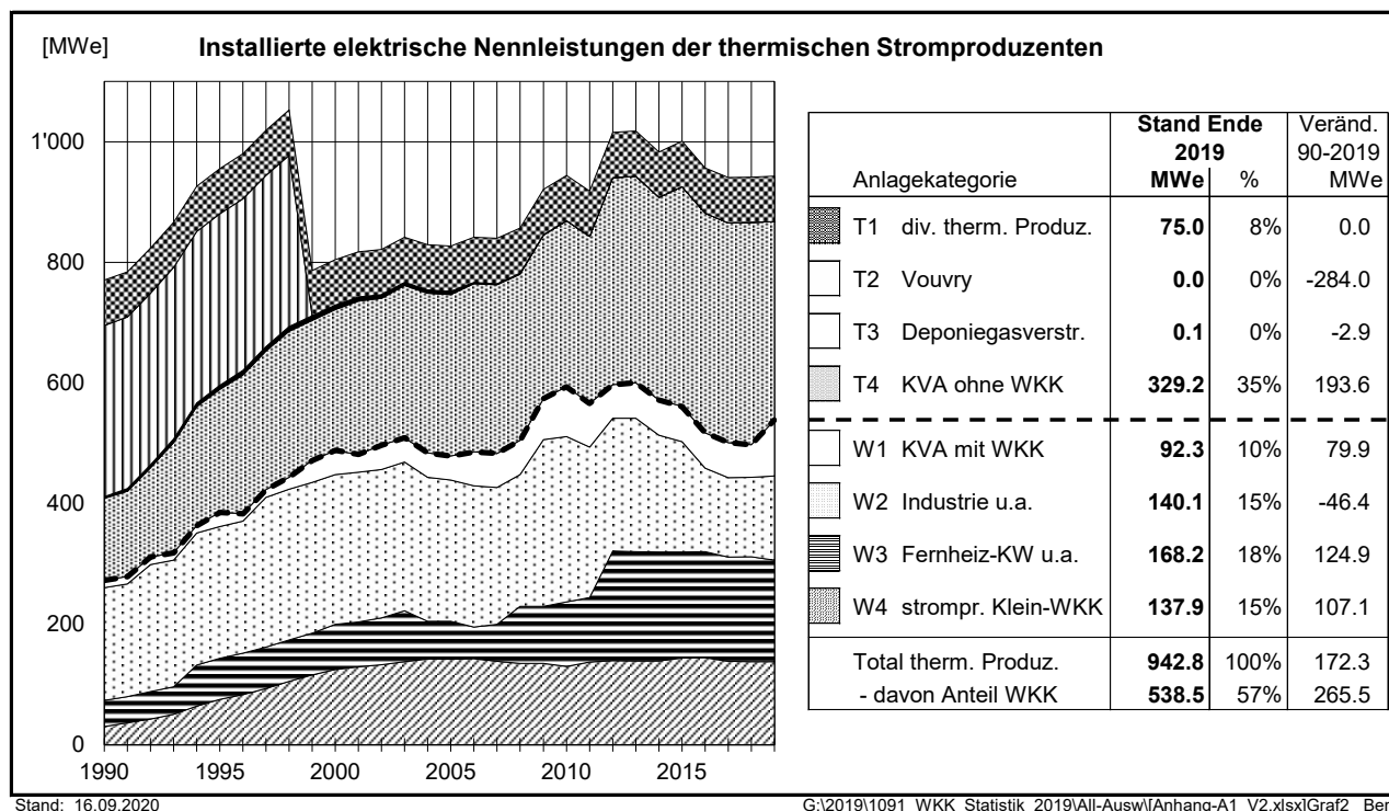
Bild 3.1b Entwicklung der installierten elektrischen Nennleistungen
