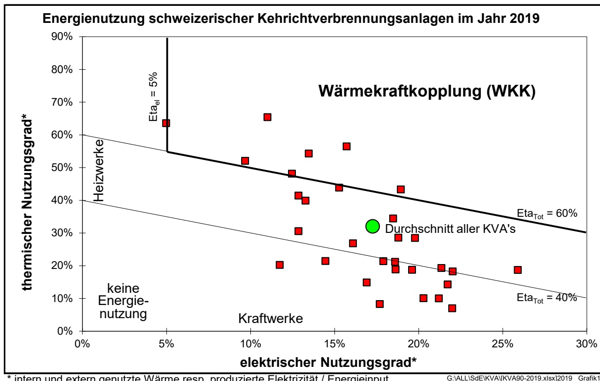
Bild 2.3 Jahresnutzungsgrade der schweizerischen Kehrichtverbrennungsanlagen im Jahr 2019
